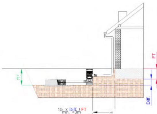
2. ábra: Telepítési helyzet: A szikkasztó blokk mélyebben van, mint az alapzat.
