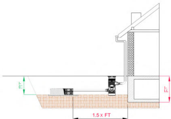
1. ábra: Telepítési helyzet: Az alapzat mélyebben van, mint a szikkasztó blokk.
